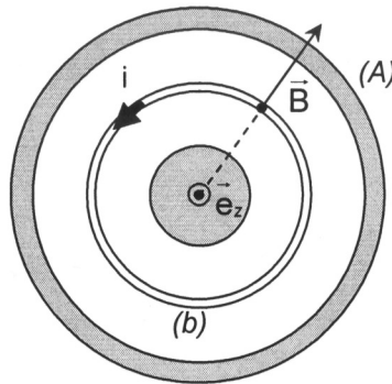
Figure 11 : Entrefer et bobine (orientation)
