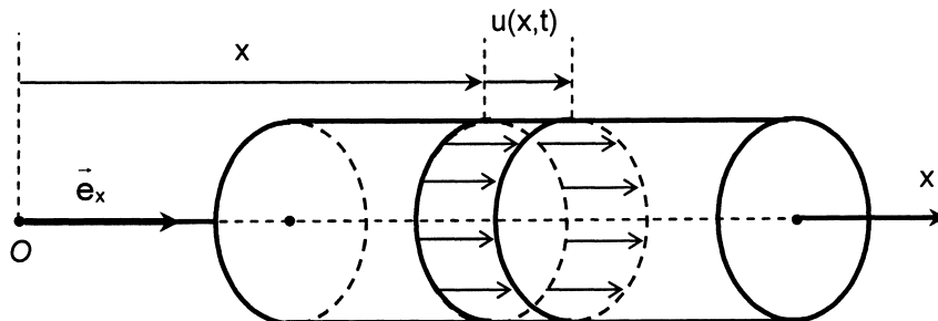
Figure 3 : Onde élastique longitudinale dans un barreau
