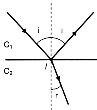
Figure 4 : Lois de Snell – Descartes
