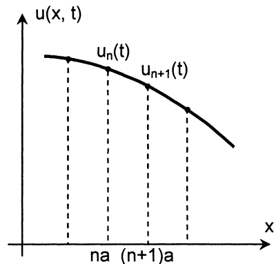
Figure 2 : Représentation de u(x, t) à t fixé
