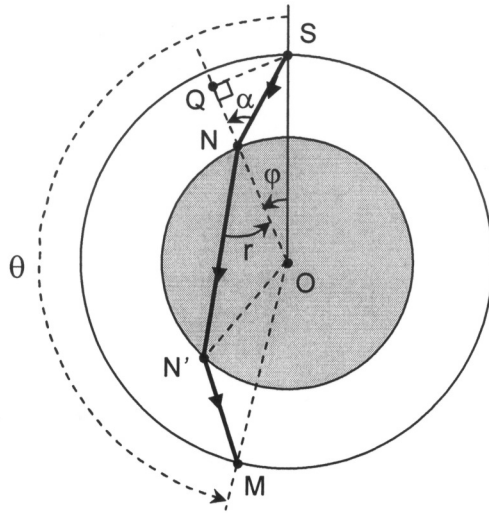
Figure 8 : Trajet du rayon réfracté
