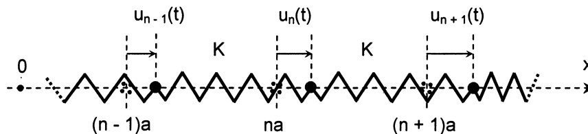
Figure 1 : Chaîne infinie d'atomes
