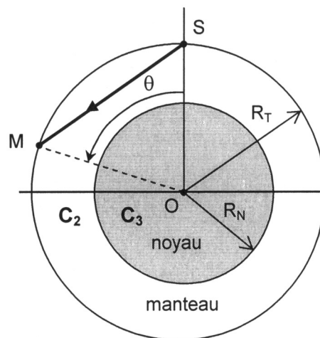
Figure 7 : Noyau et manteau terrestres
