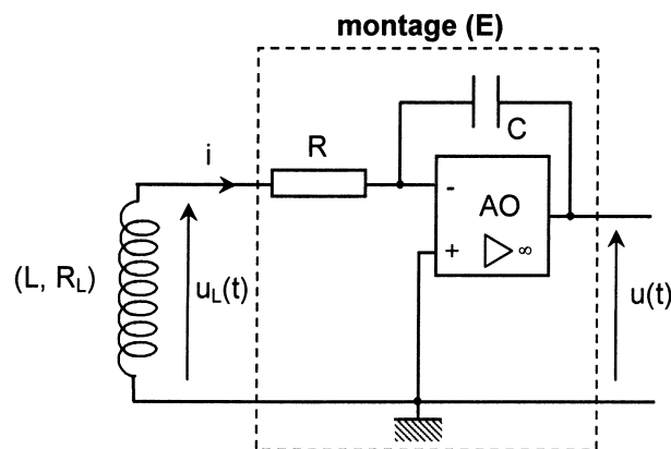
Figure 12 : Montage électronique
